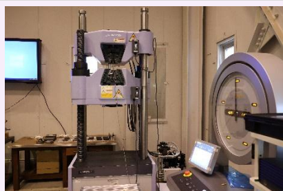
万能試験機※
